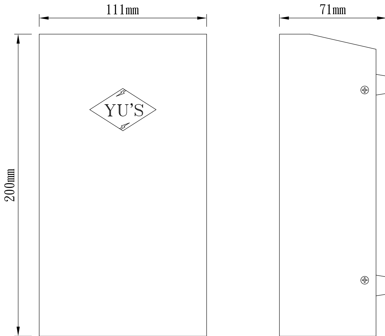
PS-13A 二線式電源主機
