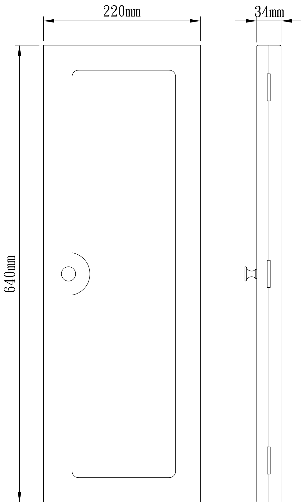
DFL 防雨箱(右開型)
