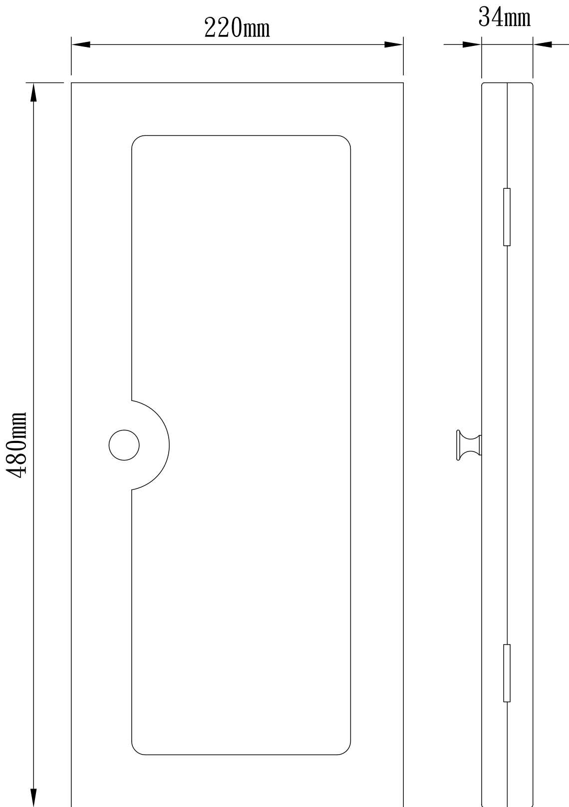
DFM 防雨箱(右開型)
