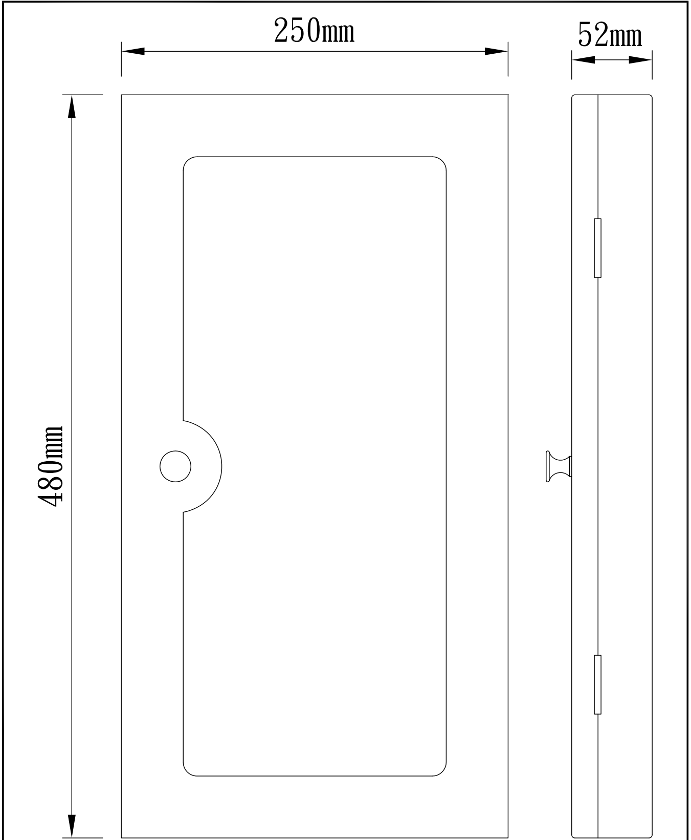
VD-11防雨箱(右開型)
