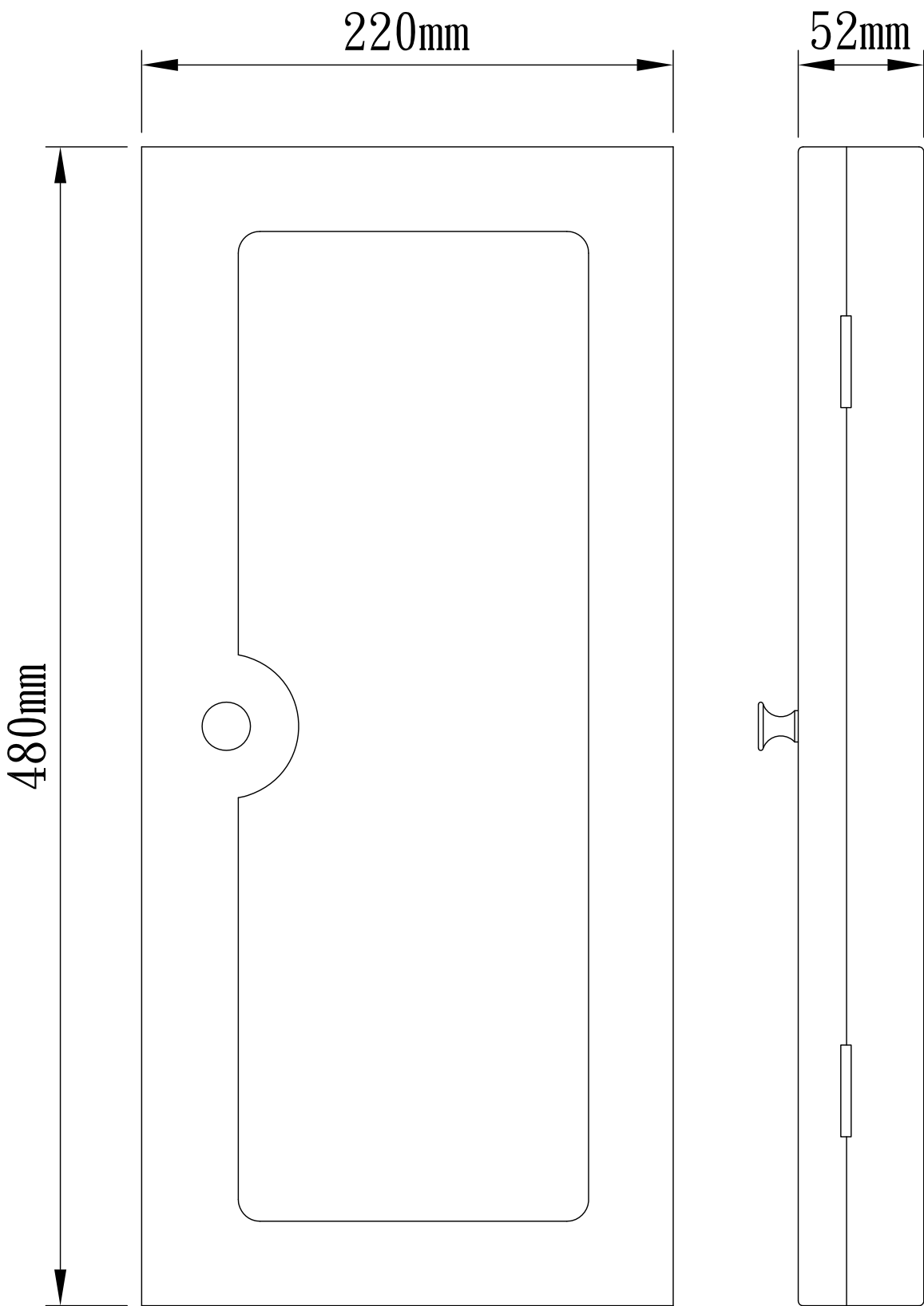
DFM掛壁式防雨箱(右開型)
