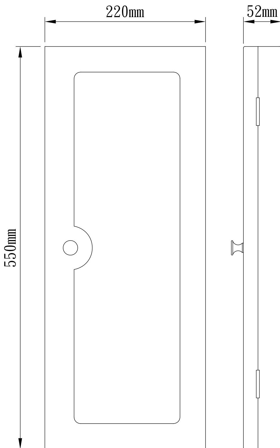
DFT掛壁式防雨箱(右開型)
