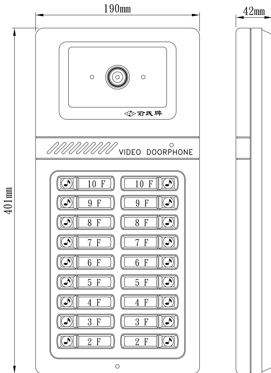
VD-13BC-18 彩色攝影門口機
